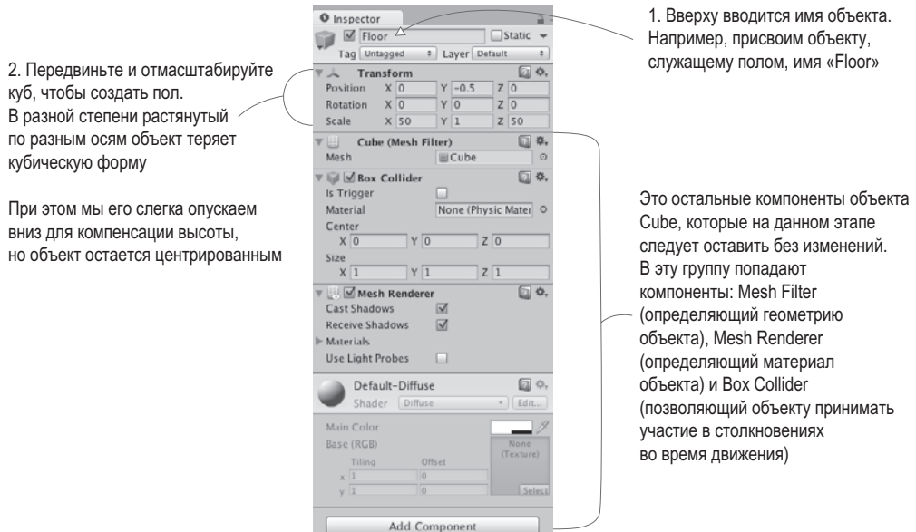
Рис. 2.6. Панель Inspector для пола
