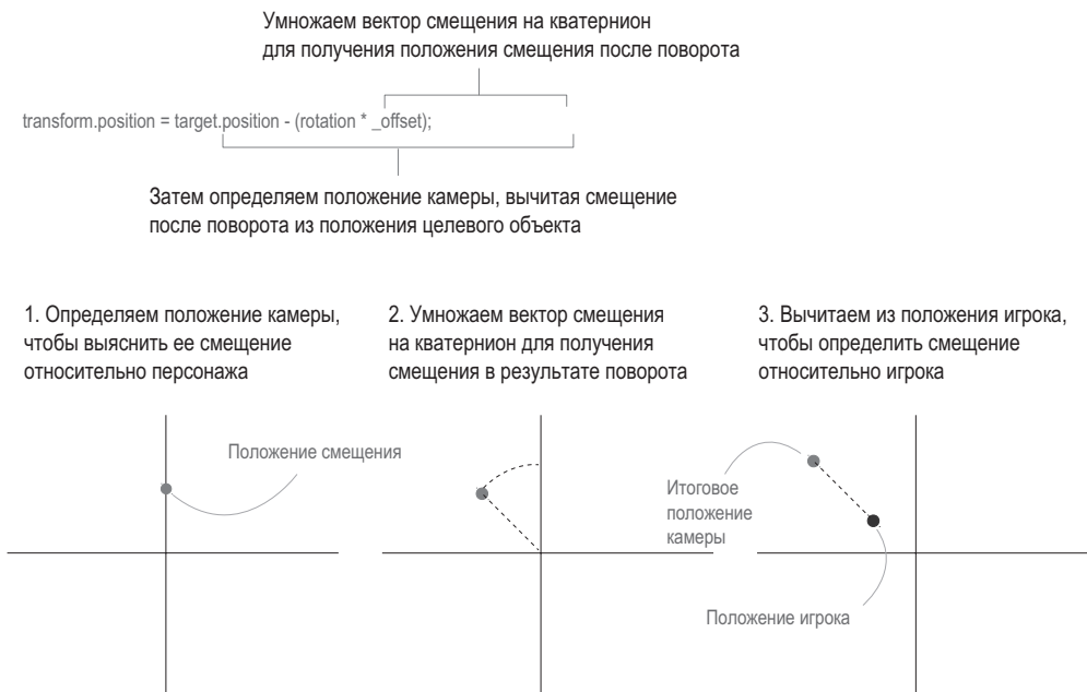
Рис. 7.7. Этапы вычисления положения камеры
